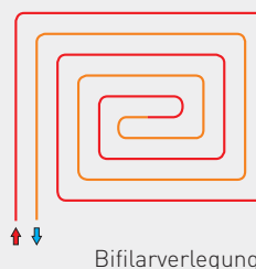
Bifilarverlegung
