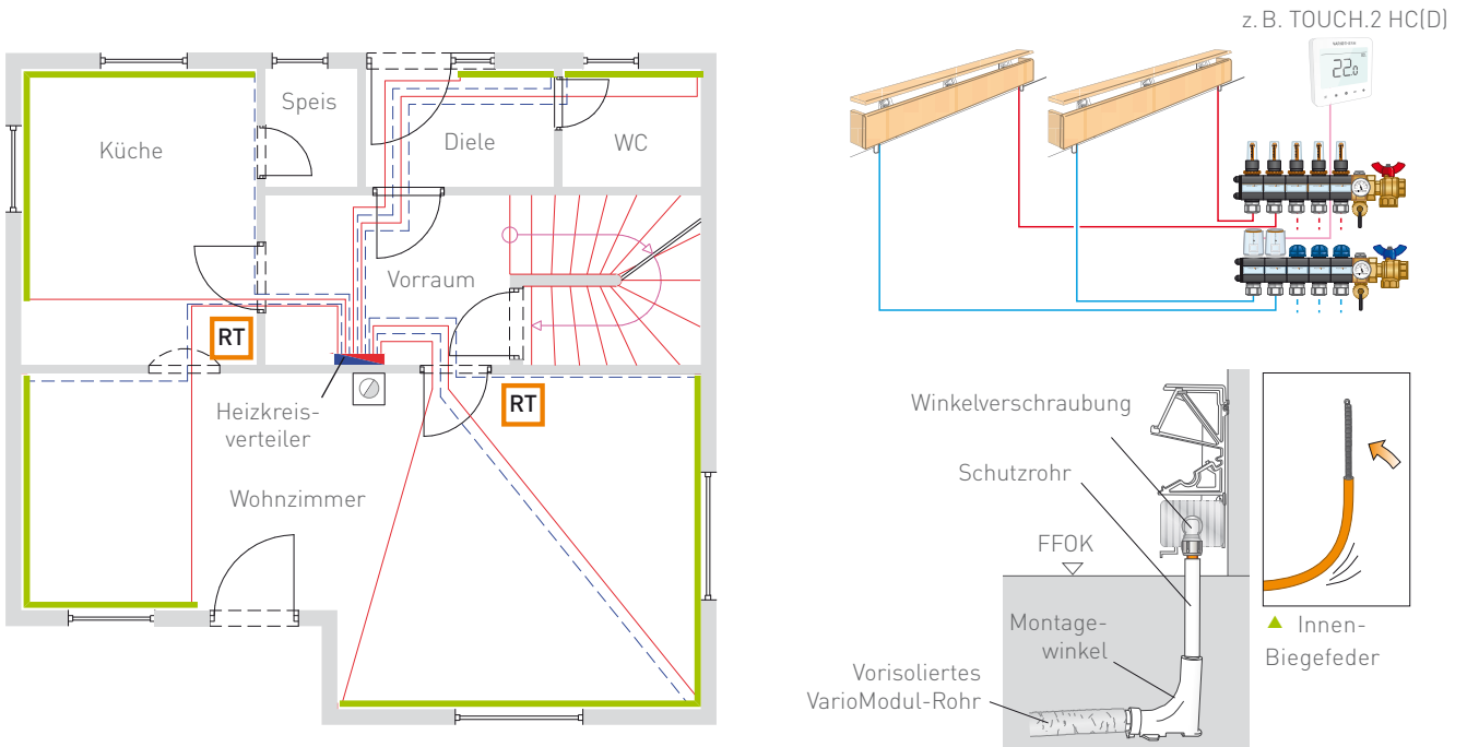
▲ Verlegebeispiel mit Variotherm Heizkreisverteiler
