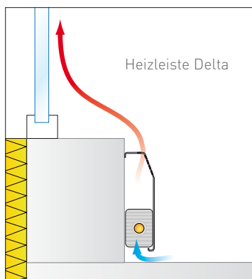
▲ Heizleisten vor Glasflächen – Schnitt
